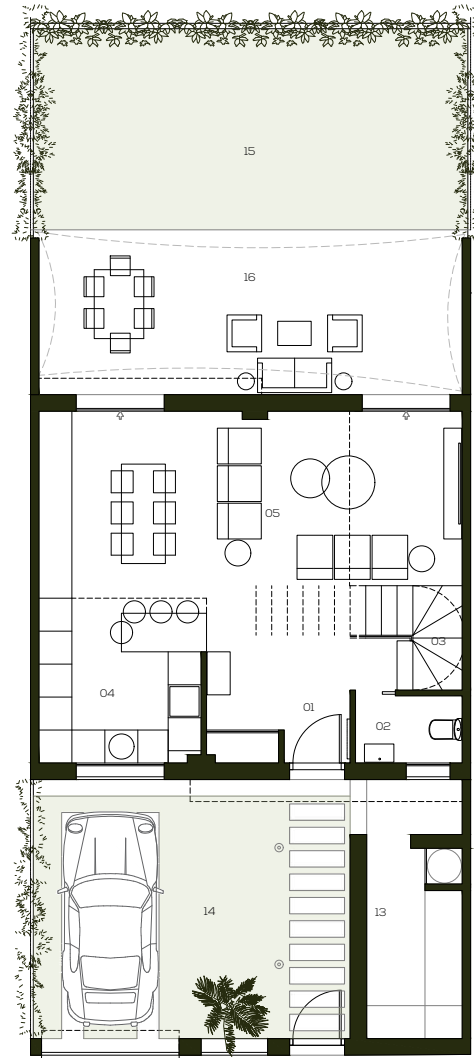
PLANTA BAJA
